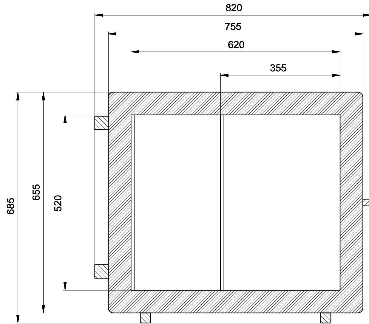
Ansicht vorne
