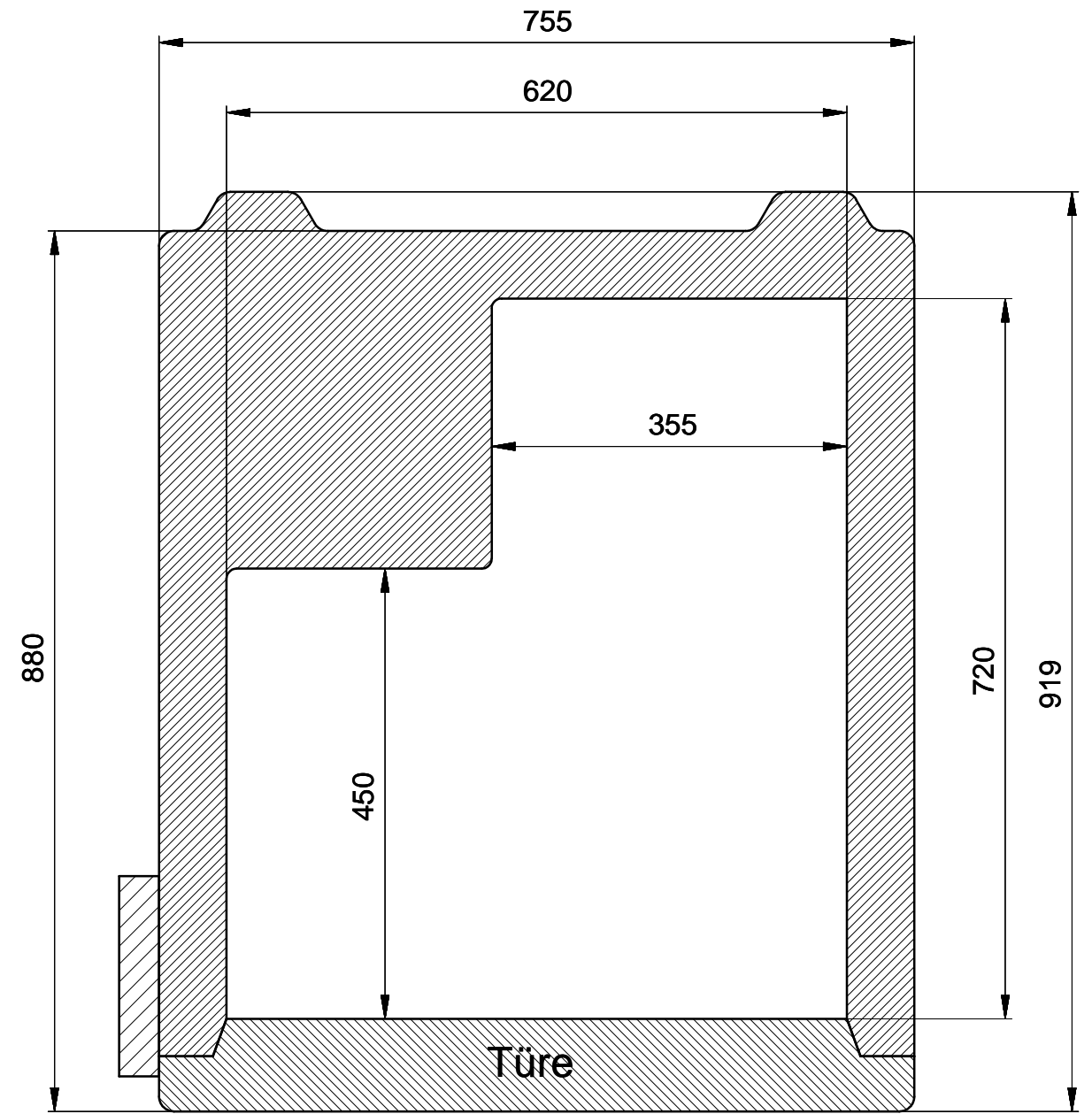
Ansicht oben
